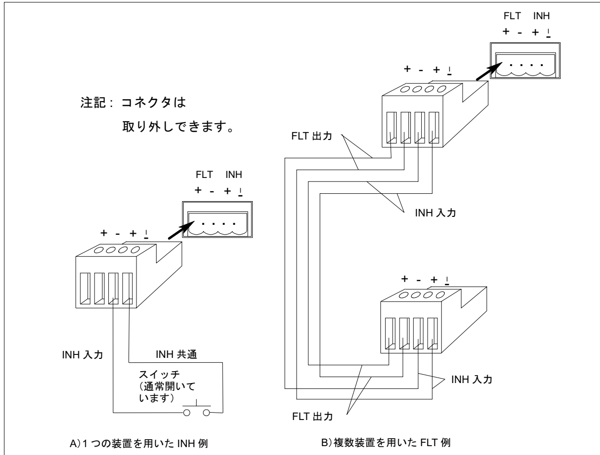
図2-6. FLT/INHの例
