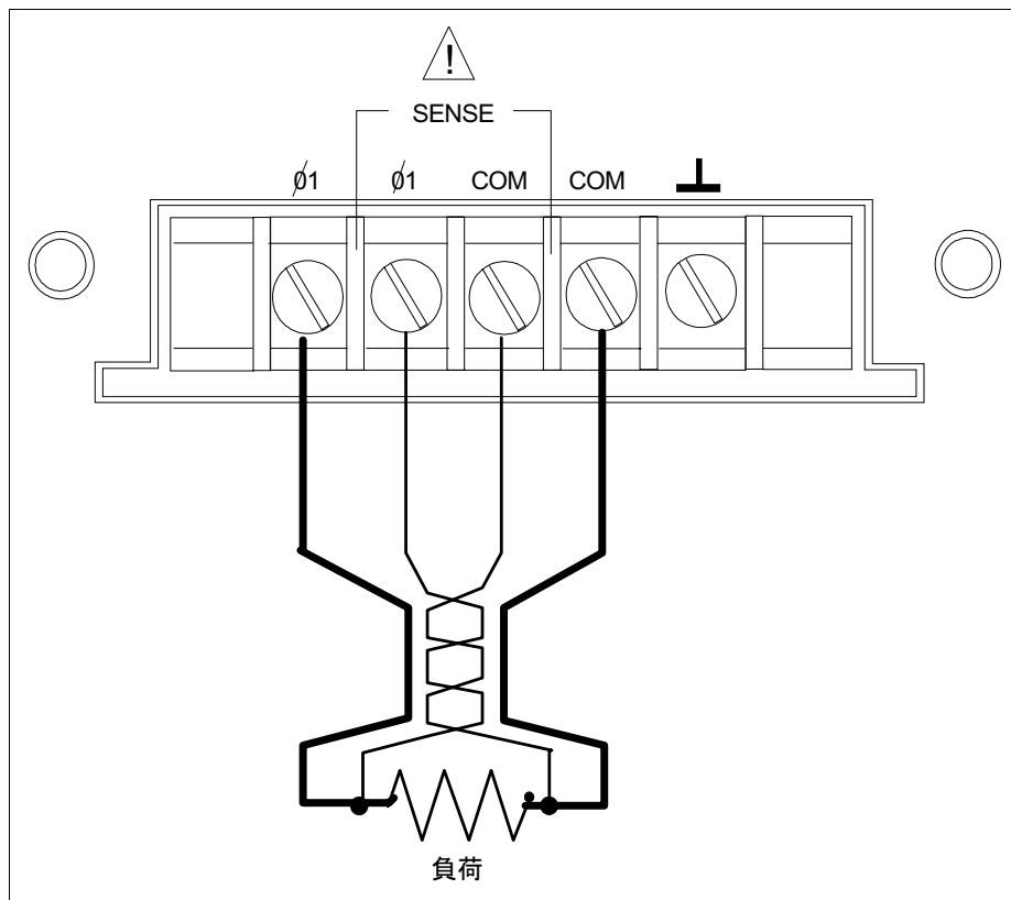
図2-5. リモート・センス接続
