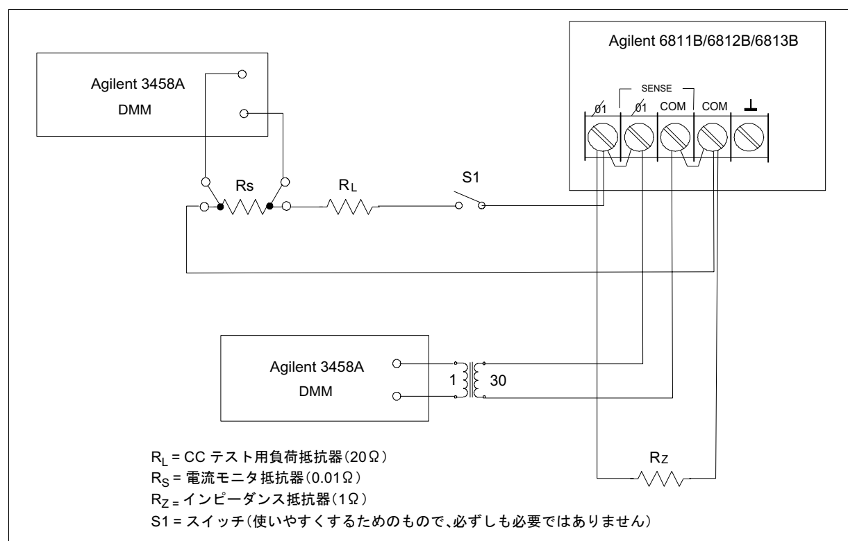
図B-1. 検査および校正テストのセットアップ
