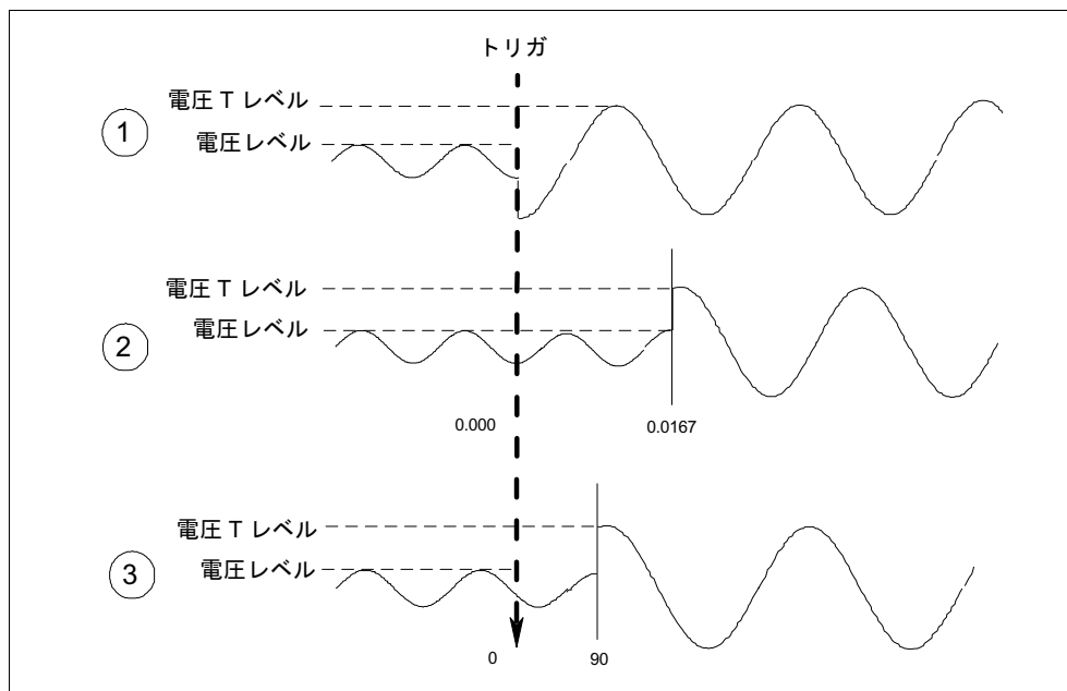
図4-7. トリガ遅延と位相の同期化
