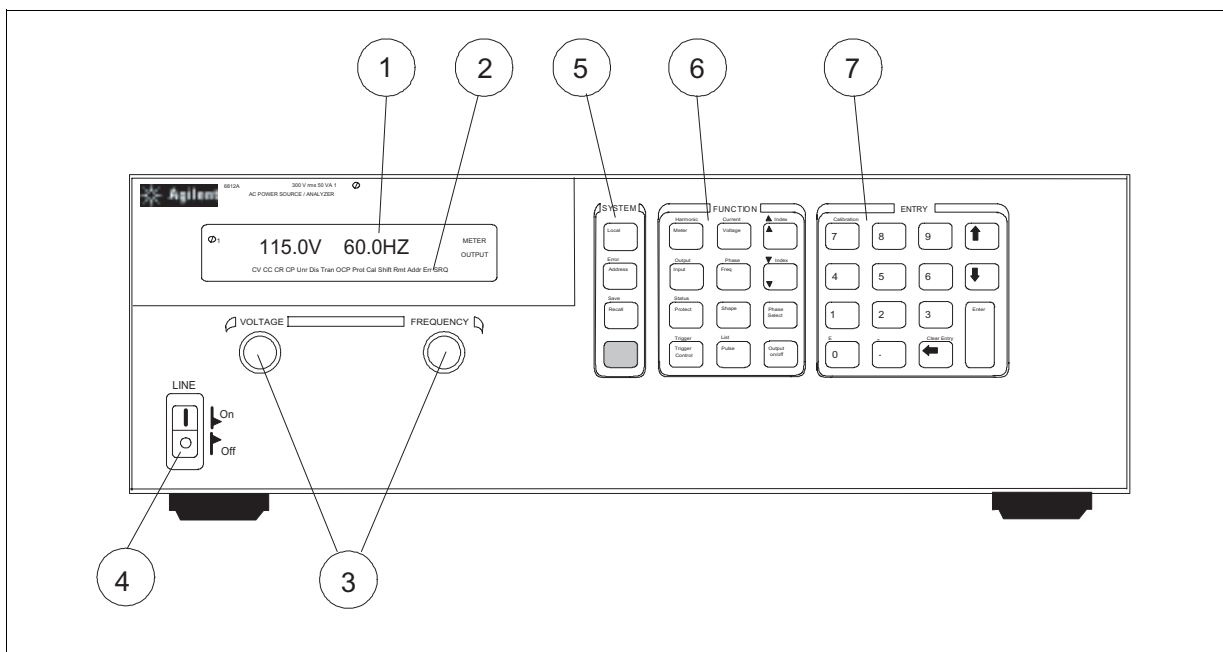
図4-1. フロントパネル外観
