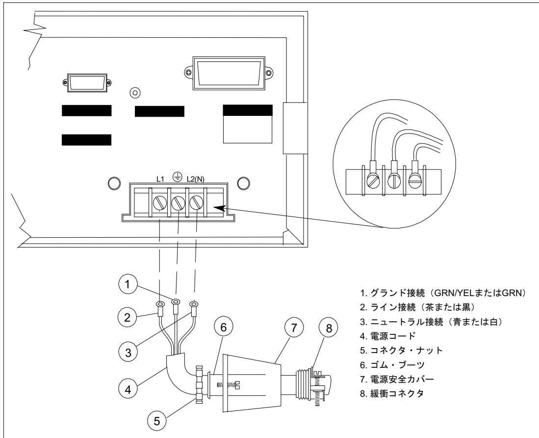
図2-3. 電源コードの接続
