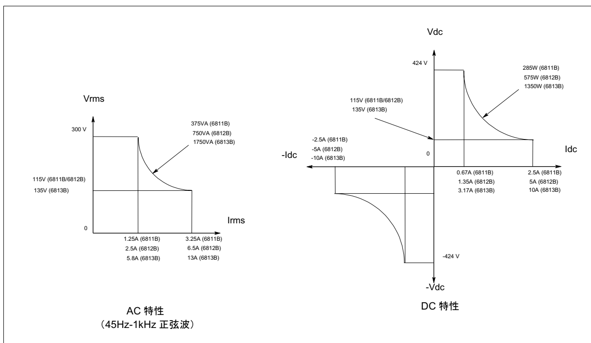
図1-2. 定常状態出力特性
