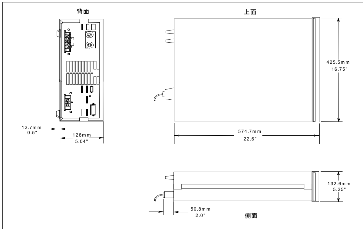
図2-1. 外形図
