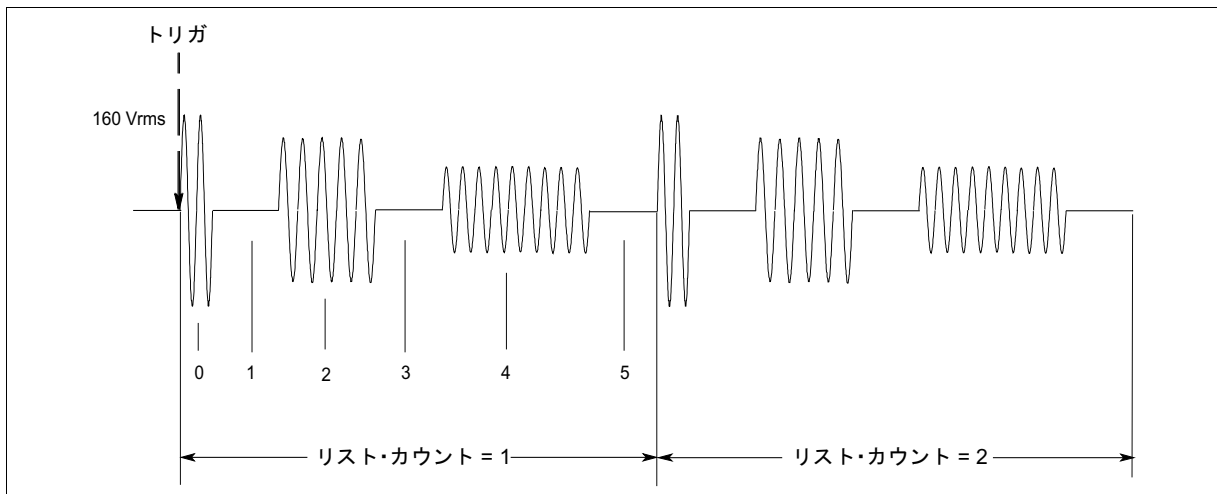
図4-6. リスト過渡信号
