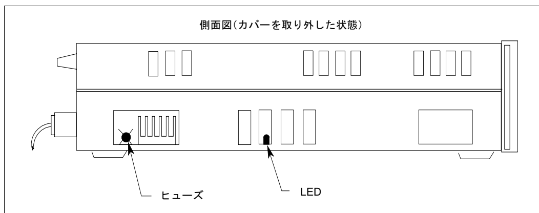
図3-2. AC電源のヒューズの位置
