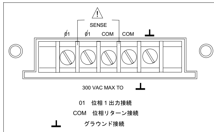
図2-4. 出力接続
