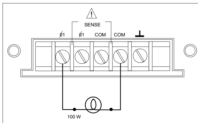
図3-1. 検査接続
