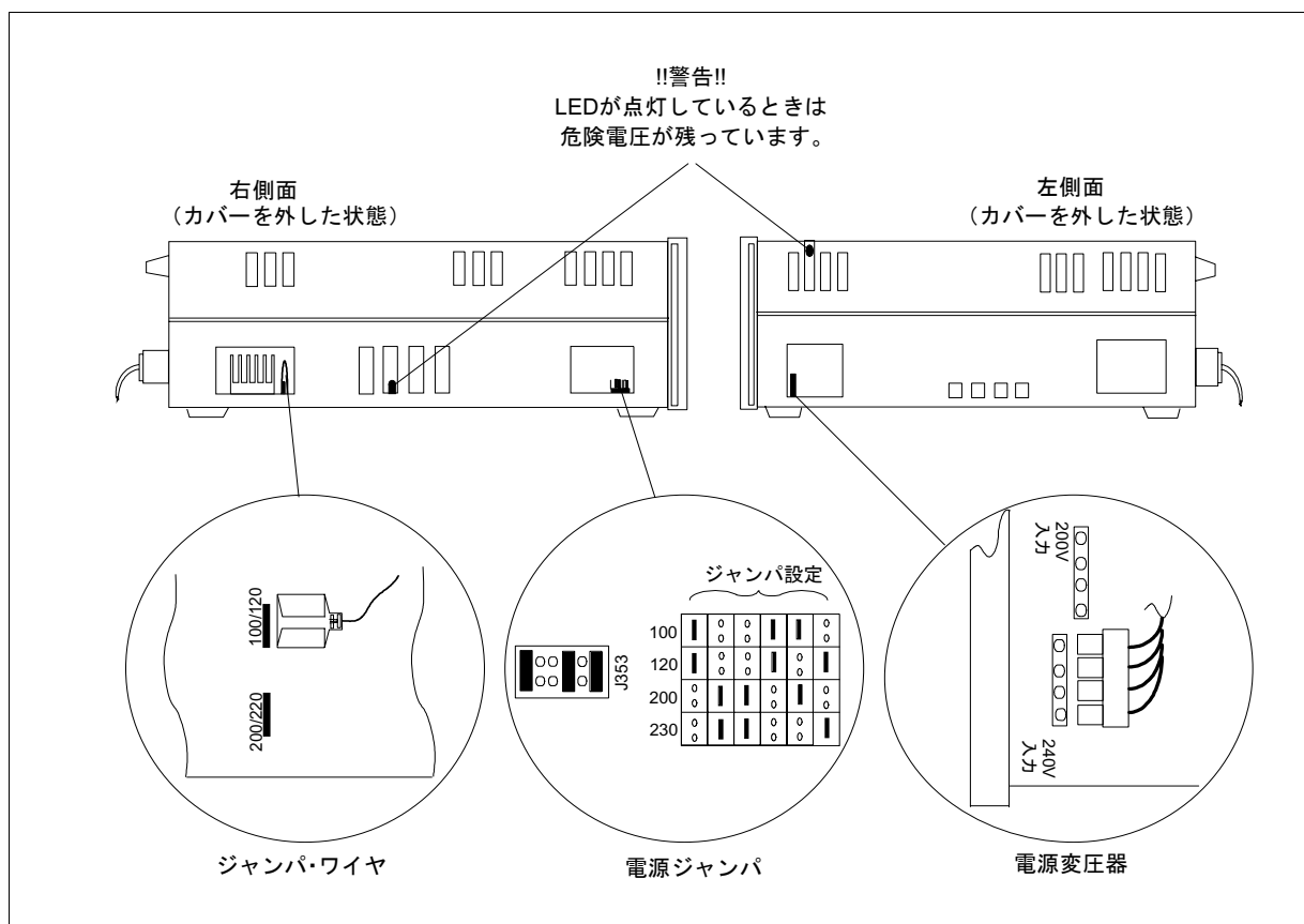
図D-1. 電源変換コンポーネント
