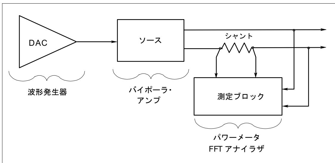
図1-1. AC電源の機能
