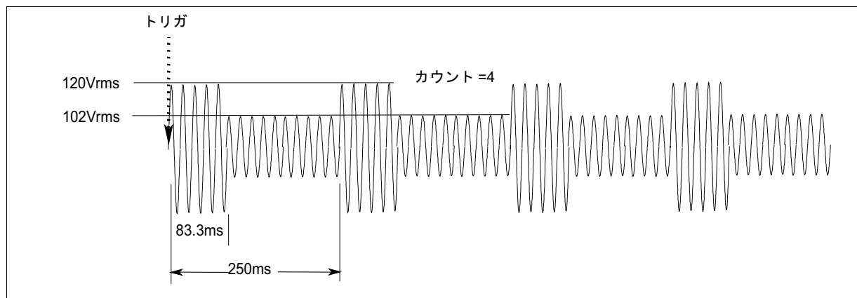
図4-5. パルス過渡信号
