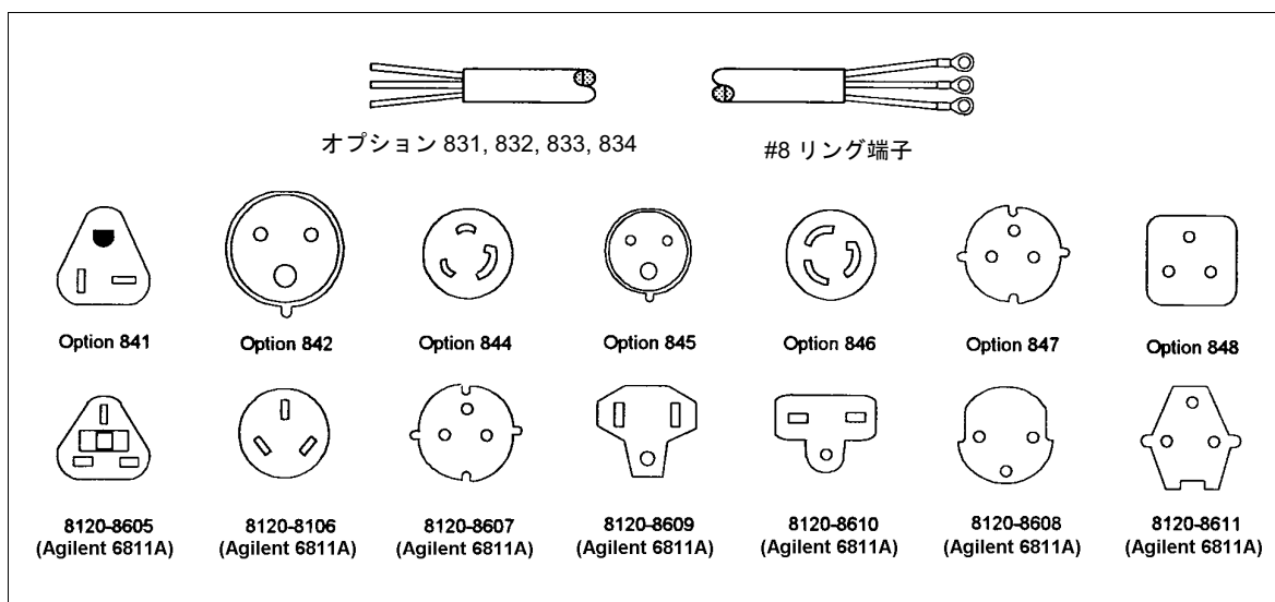
図2-2. 電源コード・プラグ構成
