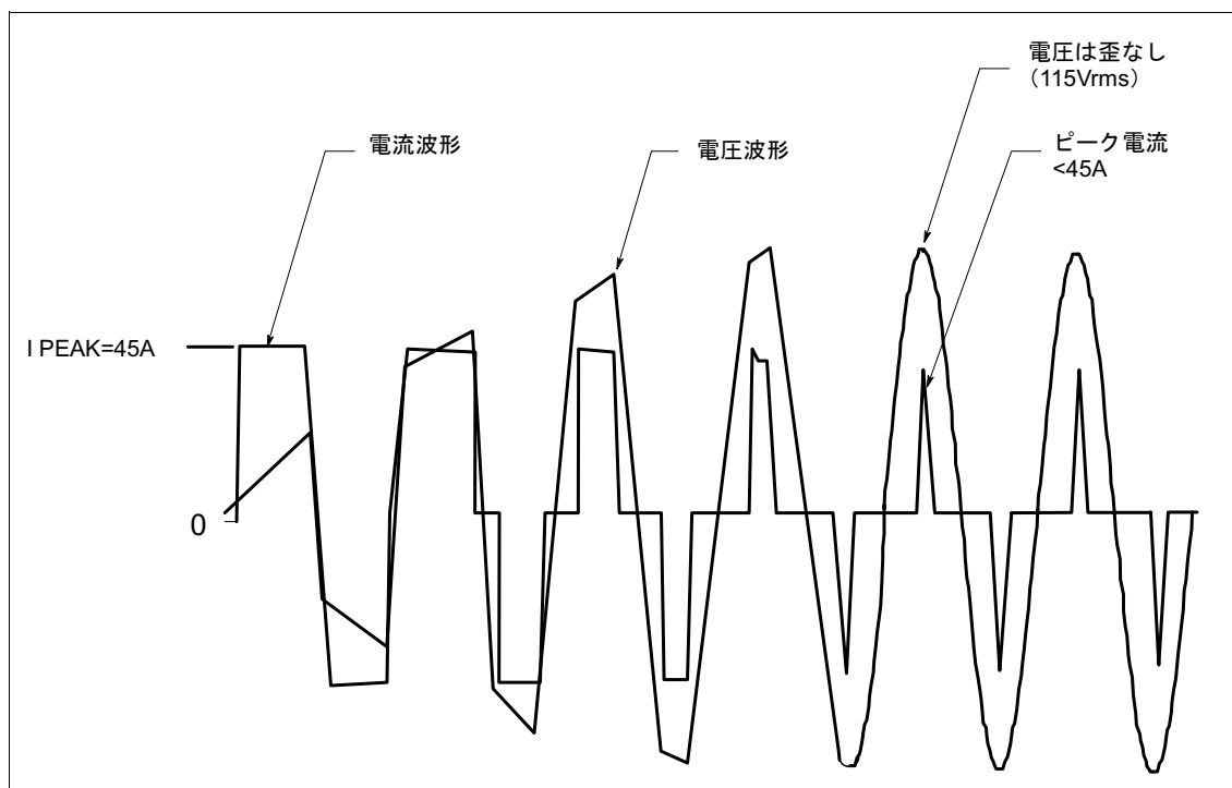
図1-3. ピーク流入電流例
