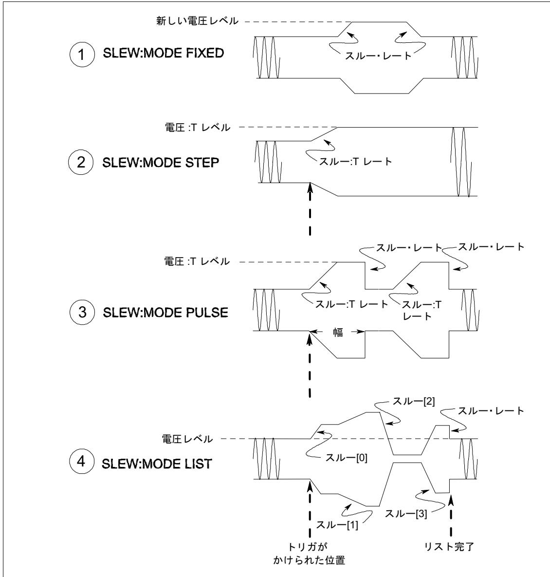
図4-8. プログラミング・スルー・レート
