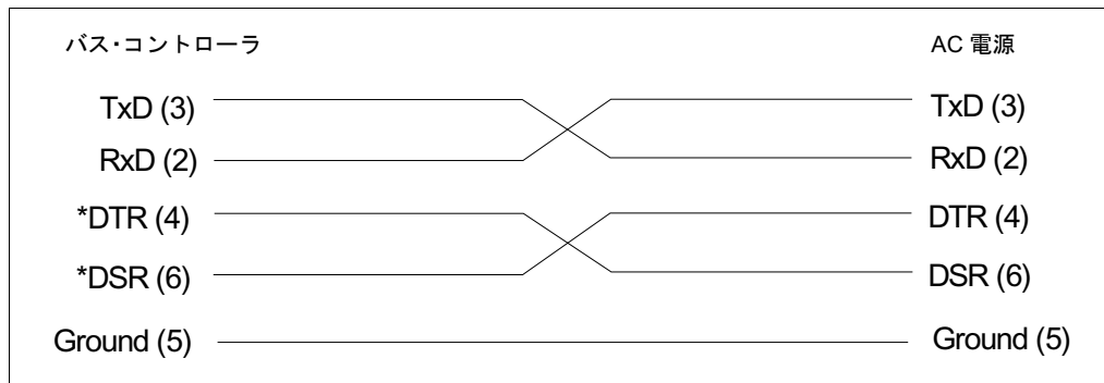
図2-7. インタフェース・ケーブル・ライン
